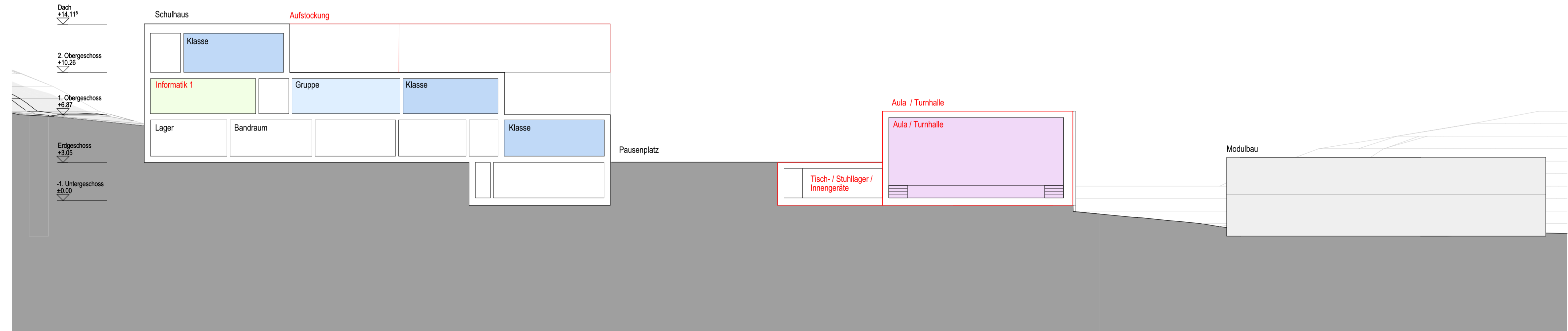
Querschnitt B-B
